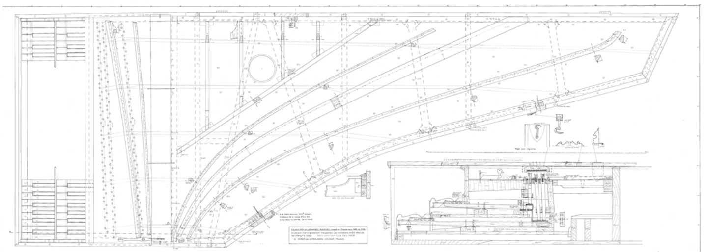
Christopher Clarke, Plan im Maßstab 1:1 des Ruckers-Cembalos von 1624, Paris, 1981, Tusche auf Transparentpapier © Musée Unterlinden, Colmar
